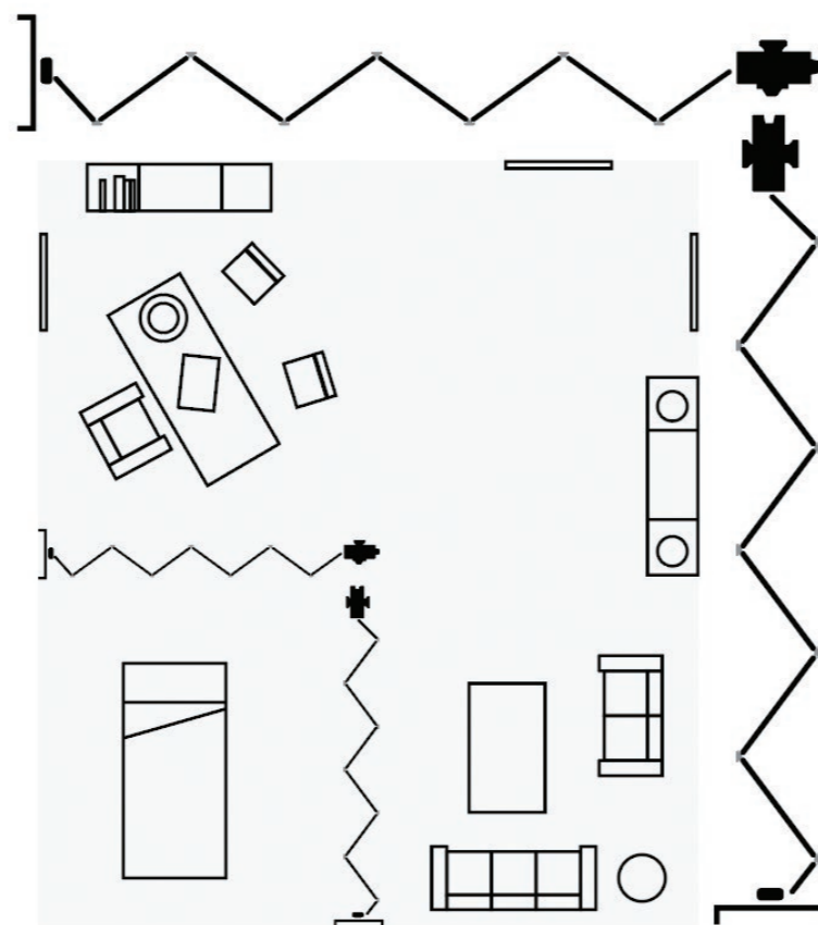
5 DOS HOJAS EN ANGULO: Consultas con camillas de oscultación, despachos, dormitorios en salones, etc.
