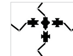
Detalle de encuentro de cuatro hojas en cruz
